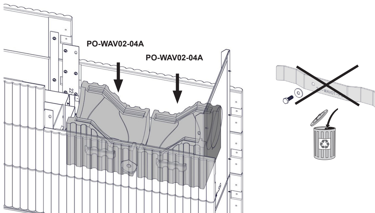
Bakre røykrørstilkobling / Bakre rökrörsanslutning Rear flue connection / Savupiippuliitântä takana Hinterer Rauchgasabschluss / Raccordement du conduit par l'arrière
