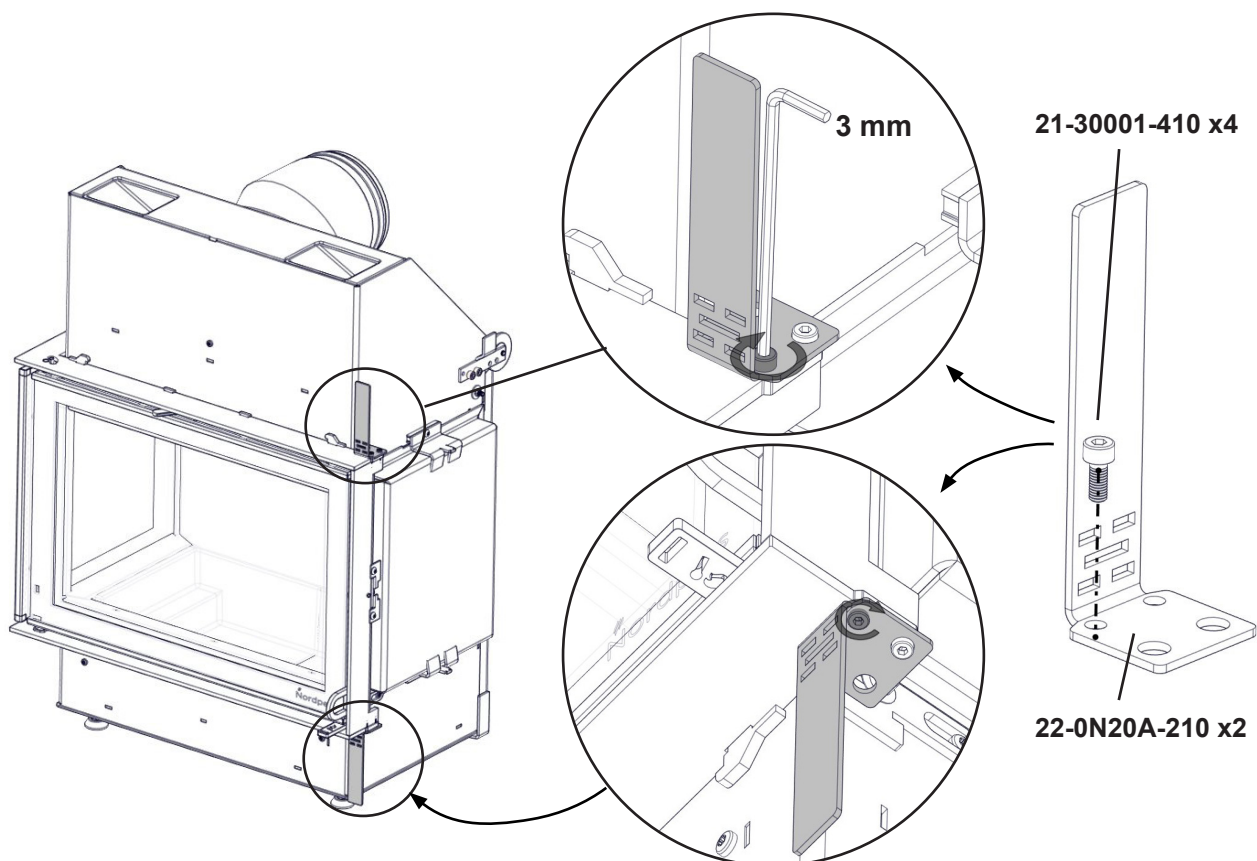
FIG 12 N-20A Monter både øvre og nedre ristbrakett / Attach both upper and lower grate supports
