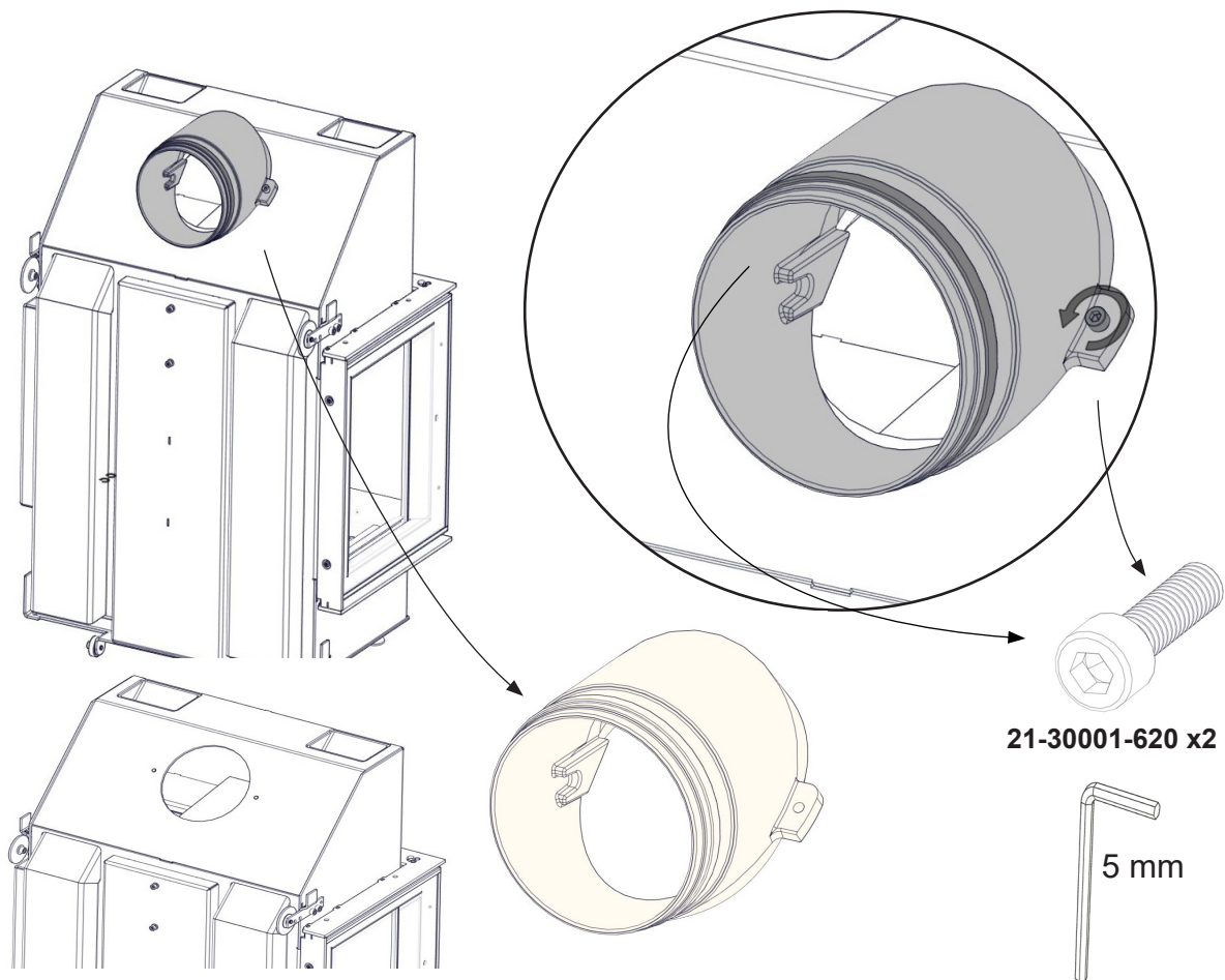
FIG 14 N-20A / N-21A Røykstussen / Chimney connection
