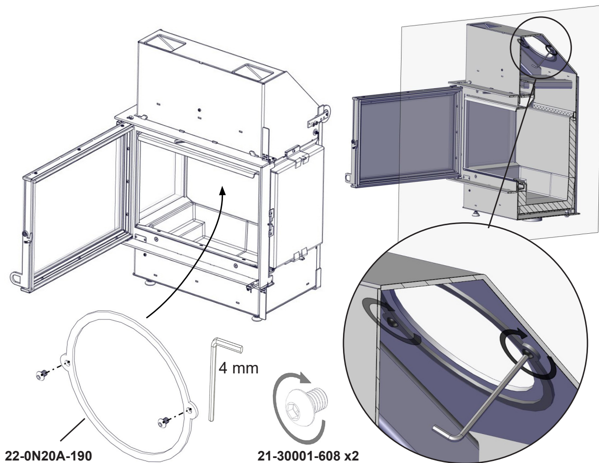
FIG 14 a N-20A / N-21A Posisjoneringsringen / Guide ring
