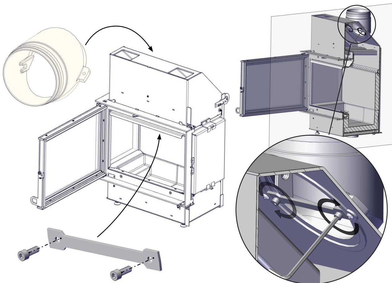
FIG 14 b N-20A / N-21A Røykstussen / Chimney connection
